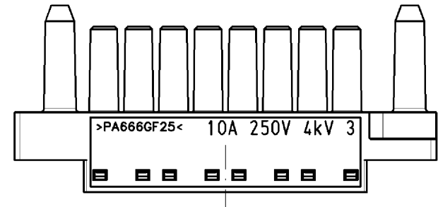
Rückansicht View back
