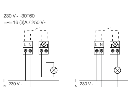
T1 POLE
